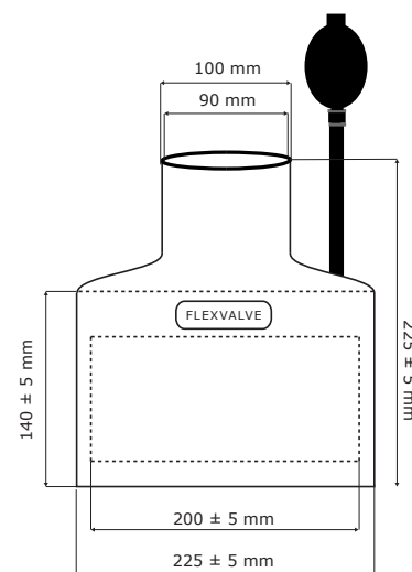
Slangetilslutning uden bøjning
