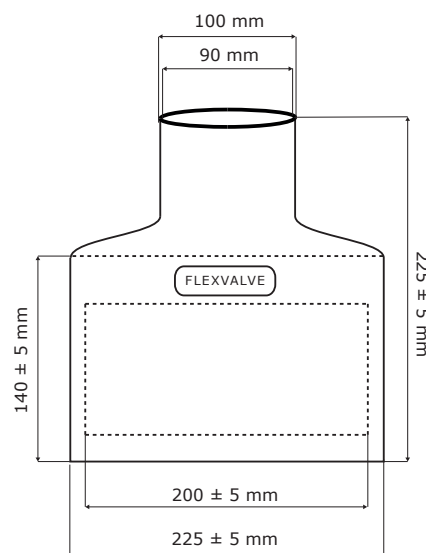
Slangetilslutning uden bøjning
