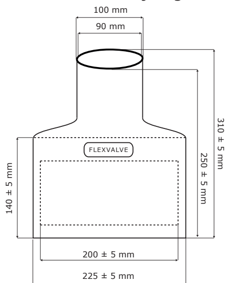
Slangetilslutning med 45° bøjning
