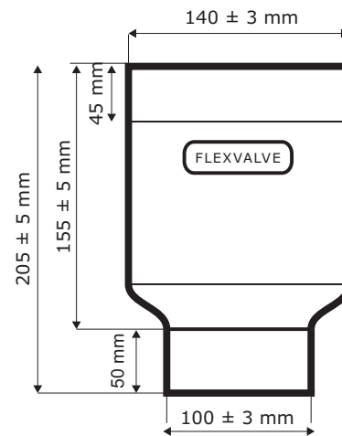
FlexGrip 4"
