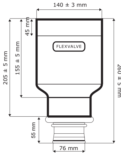
FlexGrip 3"
